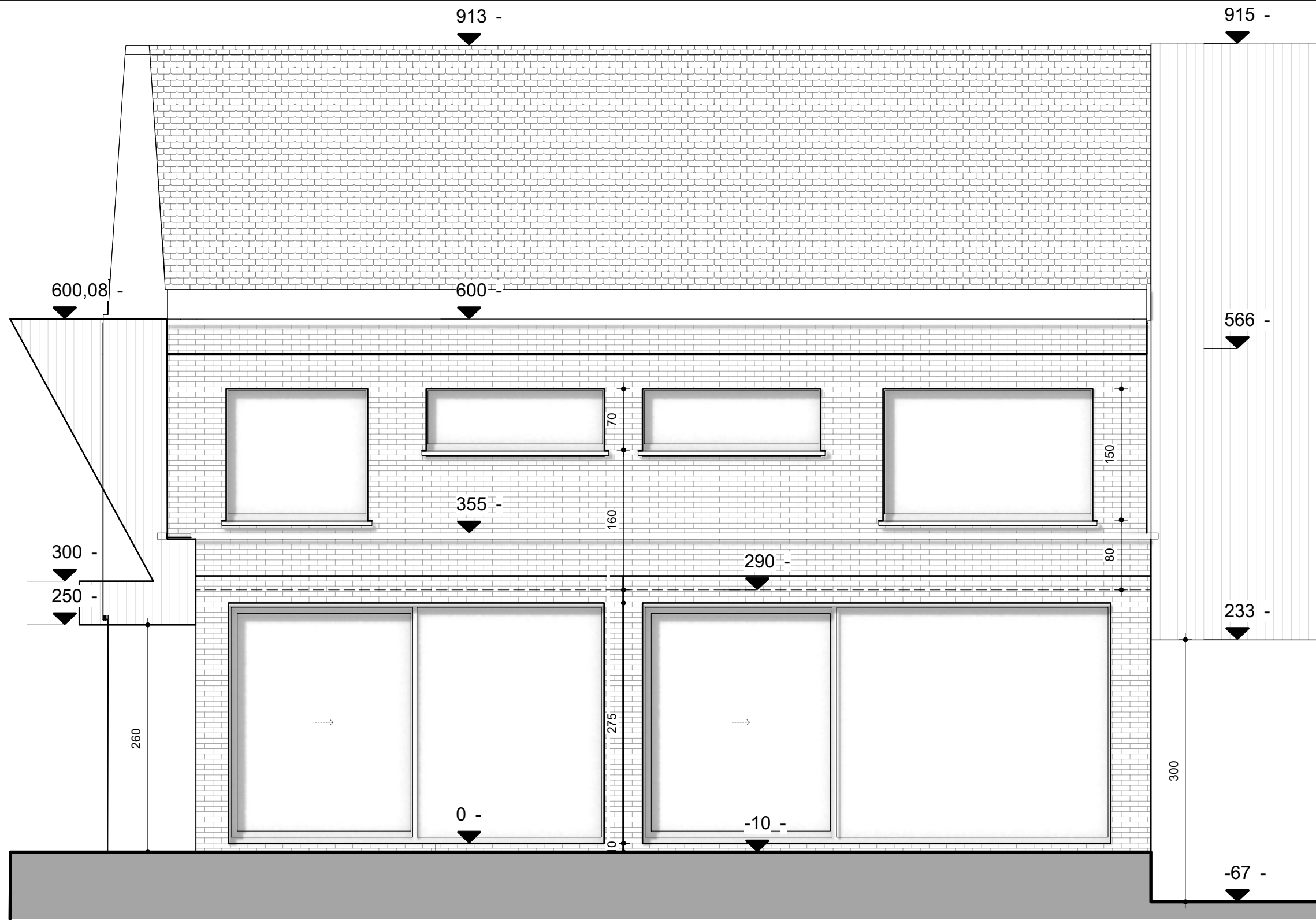
Achtergevel nieuwe toestand
